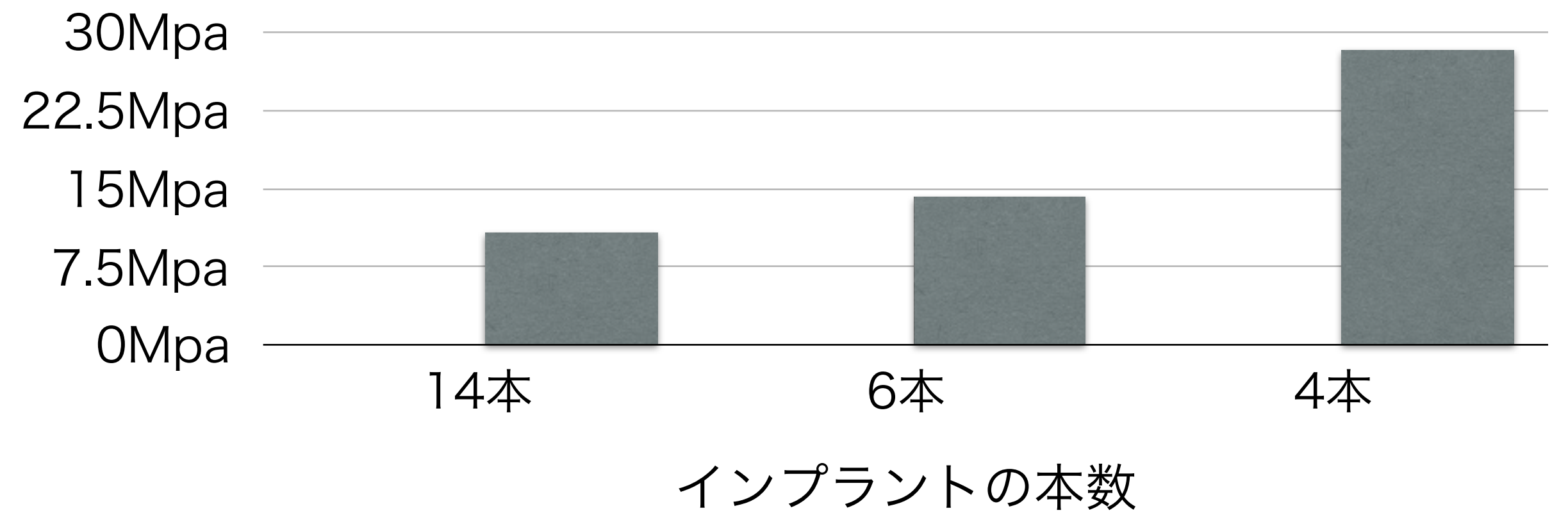
上顎インプラント1本当たりにかかる応力
